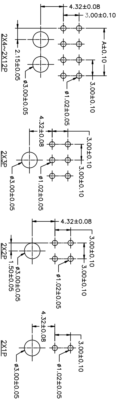
P.C.B LAYOUT
